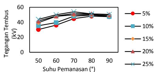
Gambar. 11. Grafik tegangan tembus minyak kelapa berbagai presentase minyak zaitun sebagai fungsi suhu pemanasan selama 90 menit.
