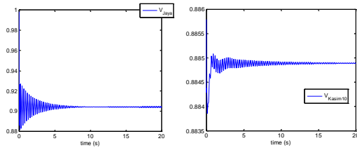
Gambar 11 Respon STATCOM pada V Jaya akibat hubung singkat
