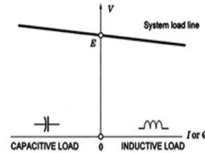
Gambar 2 Garis beban sistem
