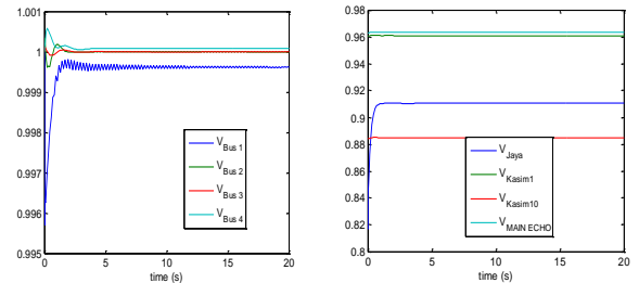
Gambar 8 Respon SVC saat starting terhadap tegangan V_{jaya} dan V_{kasim10}
