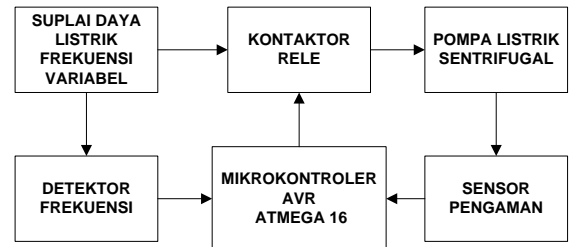
Gambar 3. Diagram blok PCU
