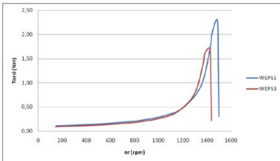
Gambar 11. Konfigurasi WEPS1 mempunyai daya output lebih besar daripada konfigurasi WEPS3
