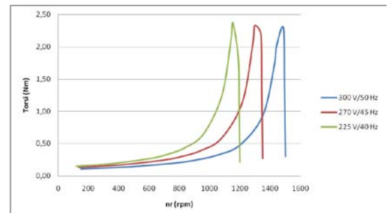
Gambar 9. Torsi output PLS dengan rasio V/f suplai (300/50, 270/45, 225/40) V/Hz
