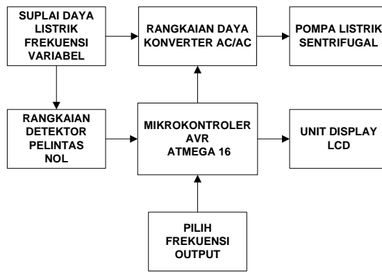
Gambar 7. Diagram blok konverter AC/AC
