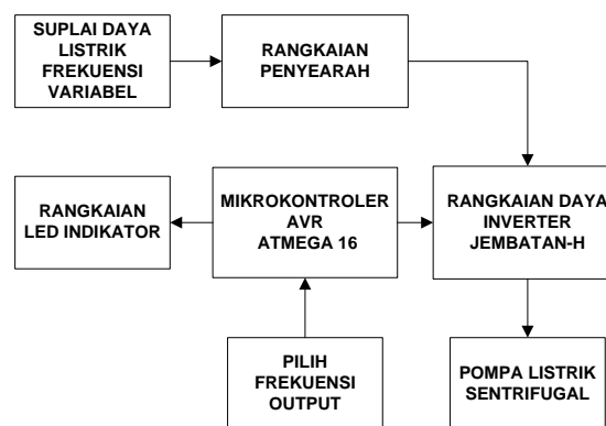
Gambar 8. Diagram blok konverter AC-DC/DC-AC
