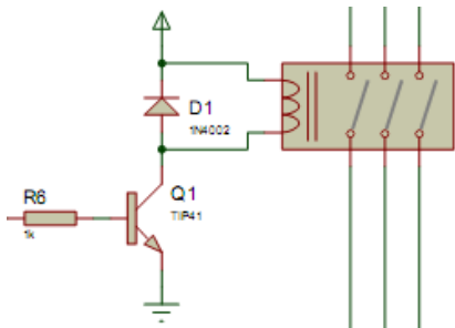
Gambar 6. Kontaktor rele dan driver input
