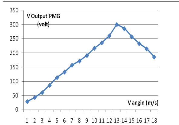
Gambar 2. Karakteristik tegangan output PMG sebagai fungsi dari kecepatan angin .
