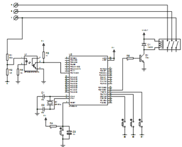
Gambar 4 Diagram rangkaian PCU
