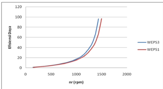
Gambar 12. Konfigurasi WEPS1 dan WEPS3 mempunyai efisiensi daya sama
