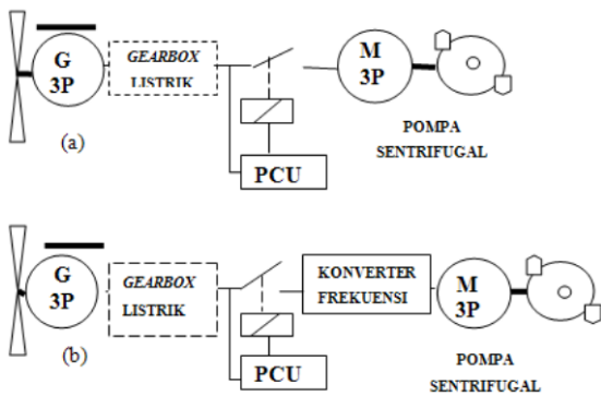
Gambar 1. Konfigurasi WEPS untuk (a) hubungan langsung dan (b) melalui konverter frekuensi.
