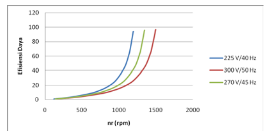
Gambar 10. Efisiensi daya PLS dengan rasio V/f suplai (300/50, 270/45, 225/40) V/Hz
